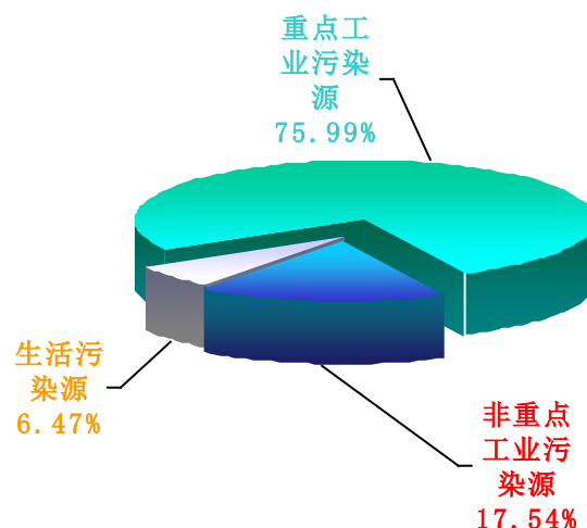
2007年二氧化硫排放总量构成比例
