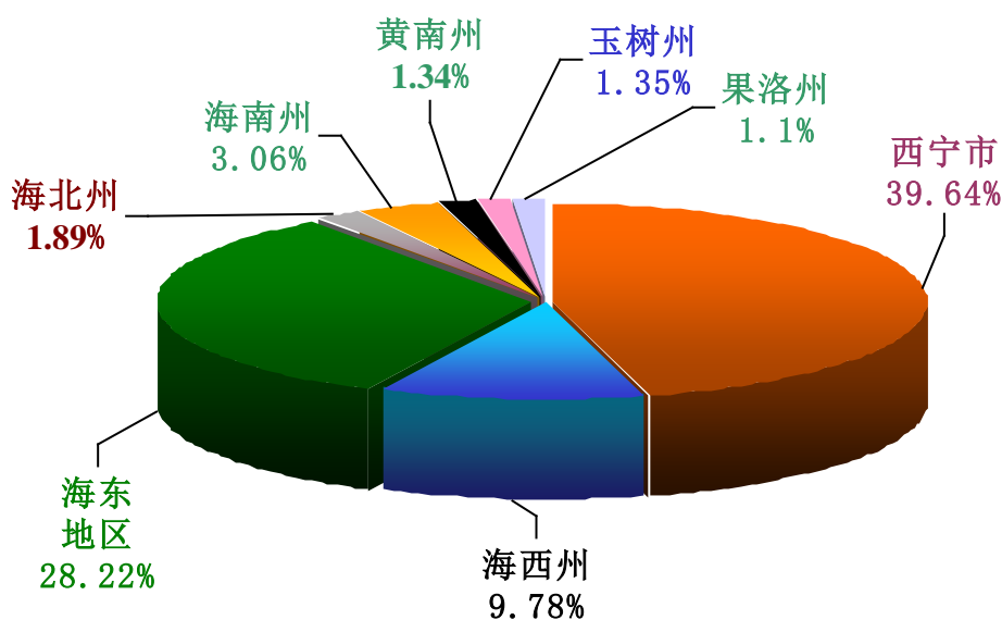
2007年各地区COD排放量占全省总量比例示意图
