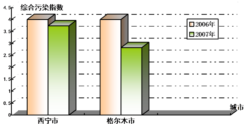
青海省城市环境空气综合污染指数历年变化图
