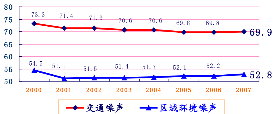
西宁市区域和交通噪声年际变化图
