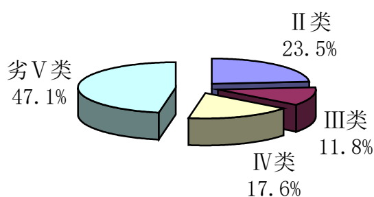
2007年湟水水系监测断面水质类别比例图
