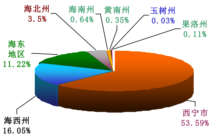
2007年全省各地区二氧化硫排放量占全省总量比例图
